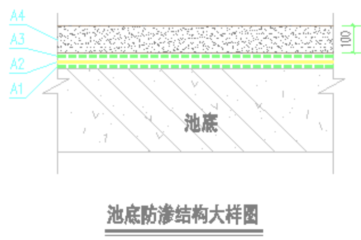
图 3. 6. 2-4 池底防渗图
