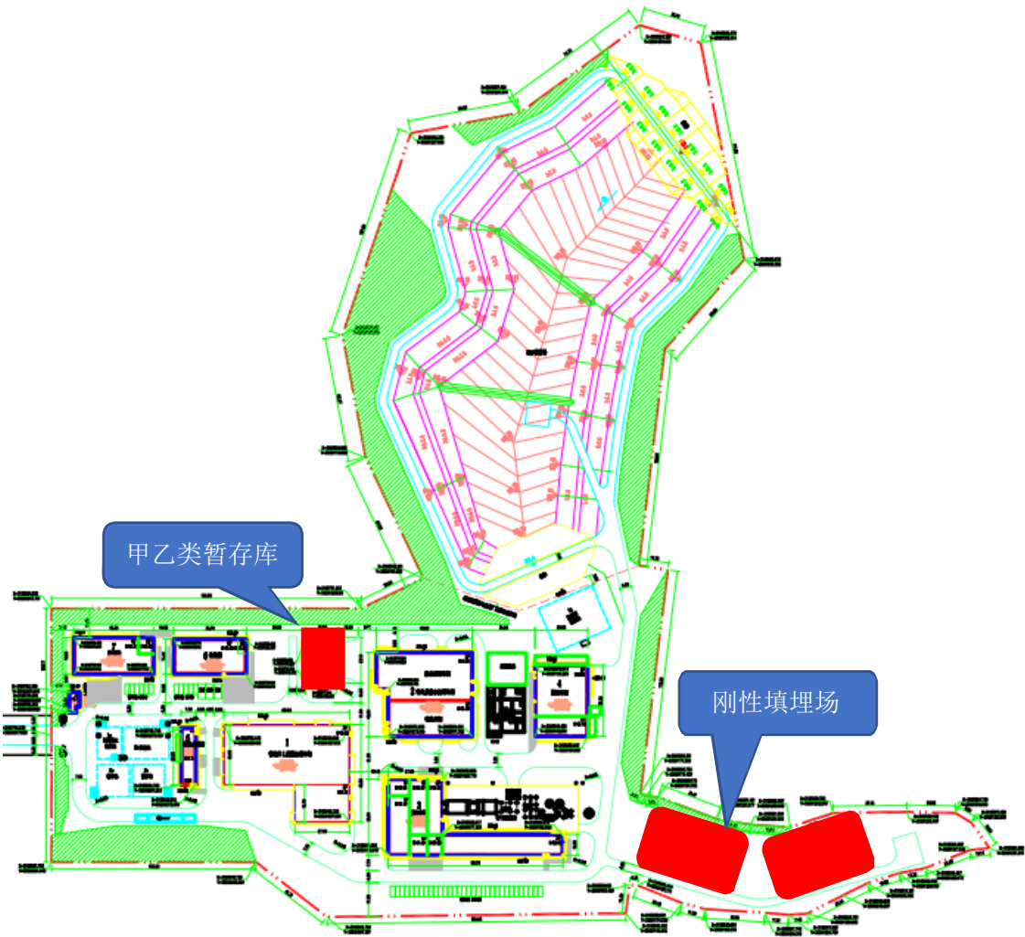
图 3.2.1-1 本次扩建方案示意图
